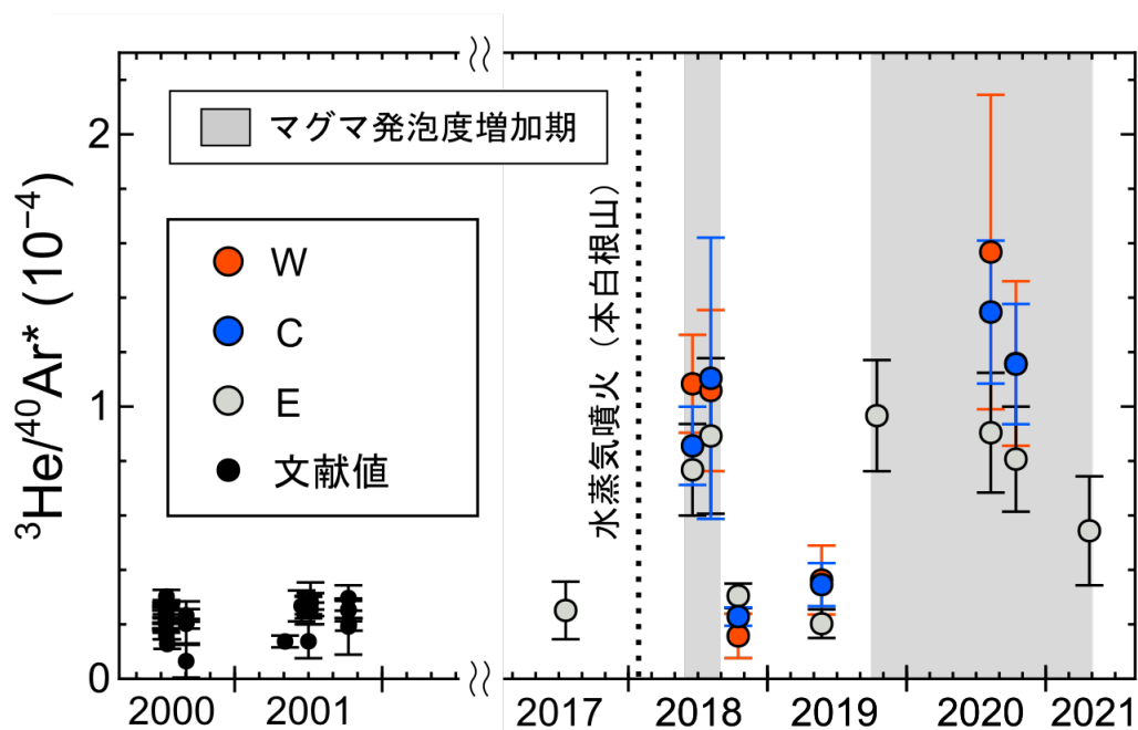
図2：草津白根山北側斜面噴気孔（W, C, E）で採取した火山ガスの ^3\text{He}/^{40}\text{Ar}^* 比の経時変化 2000 年から 2001 年にかけて同地点で採取された火山ガスの ^3\text{He}/^{40}\text{Ar}^* 比（文献値）も示して いる。網掛けで示された ^3\text{He}/^{40}\text{Ar}^* 比が高い時期にマグマ発泡度が増加していたと考えられ る。点線は 2018 年 1 月に本白根山で発生した水蒸気噴火。
