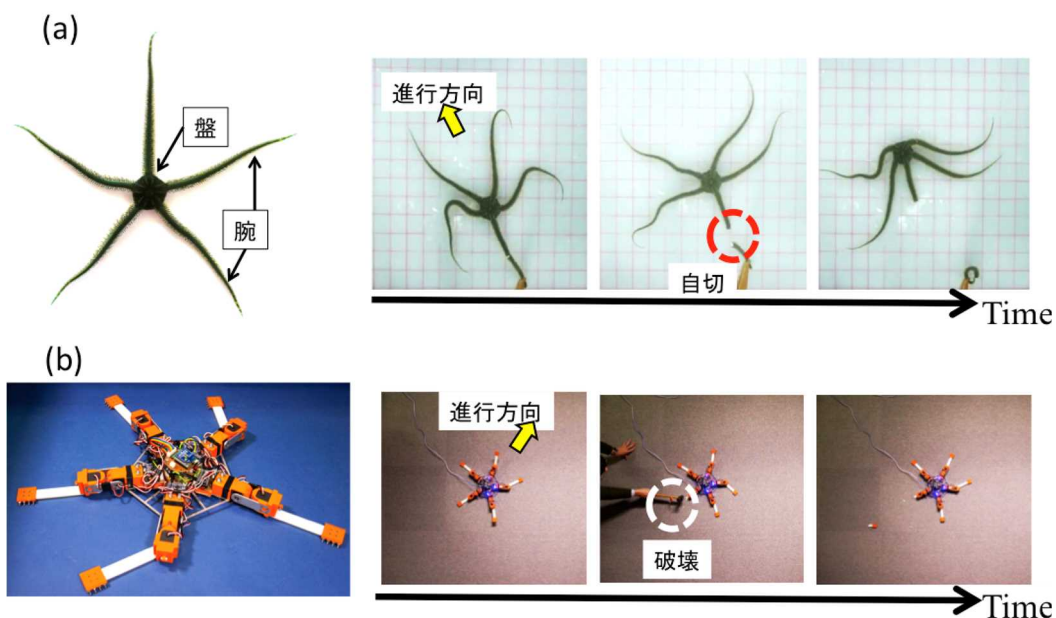
図 1 (a) クモヒトデの全体像(左)と腕を自ら切断して推進する様子(右)。(b)開発したクモヒトデ型ロボット PENTABOT II(左)と、腕を破壊した時のロボットの運動の様子(右)。ロボットの腕をいかに破壊しても即座に適応し、残った腕を協調させて推進し続けることが可能。
