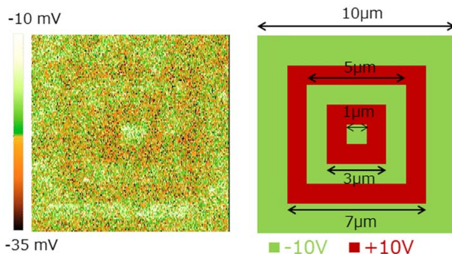
図 アンモニア気流中でポストアニールした酸窒化物ペロブスカイト SrTaO 2 N セラミックス表面を、右の電極パターン±10V で分極したのちに観察された圧電応答顕微鏡像（左）
