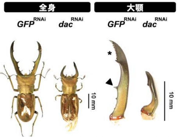
図3. dachshund 遺伝子の機能阻害による表現型
