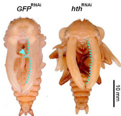
図5. homothorax 遺伝子の機能阻害による表現型
