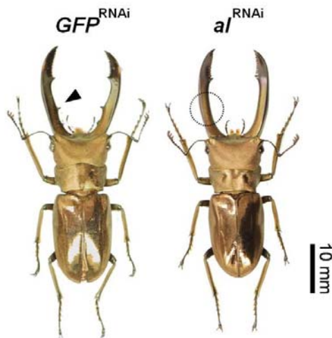
図4. aristalless 遺伝子の機能阻害による表現型
